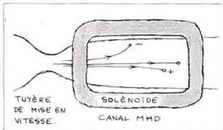
Trajectoires des particules chargées.
